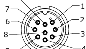
FACE VIEW P/N: 3280-9SG-5XXW
